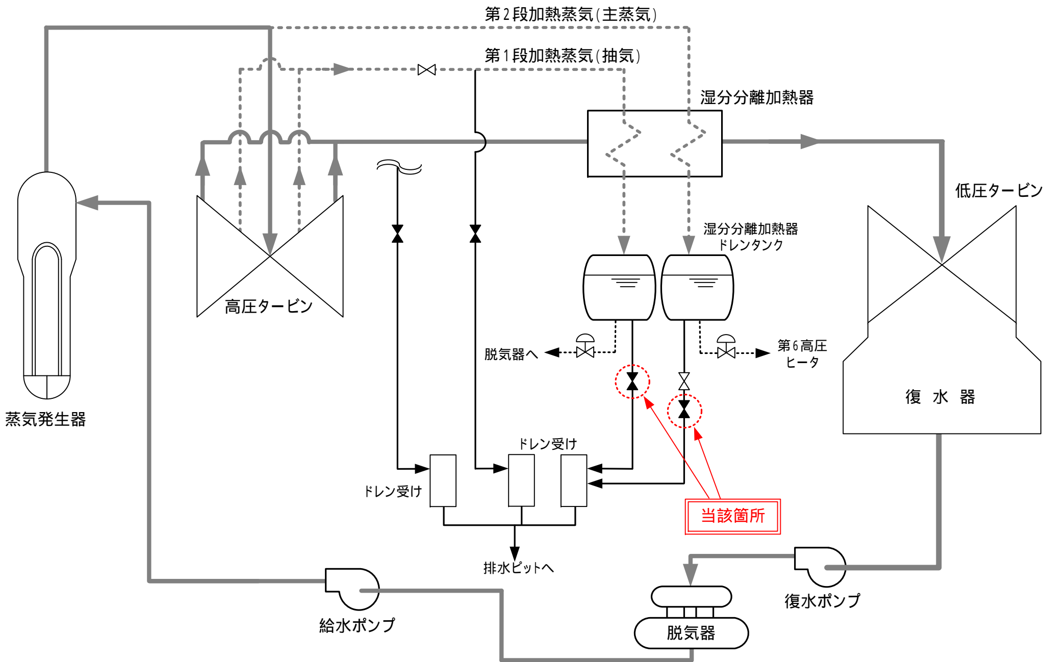
伊方発電所3号機 湿分分離加熱器まわり概略系統図
