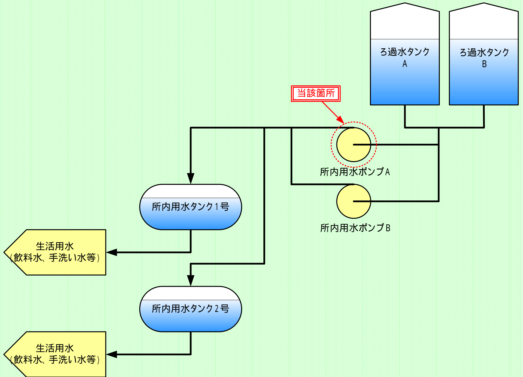
伊方発電所1、2号機 所内用水ポンプまわり概略系統図
