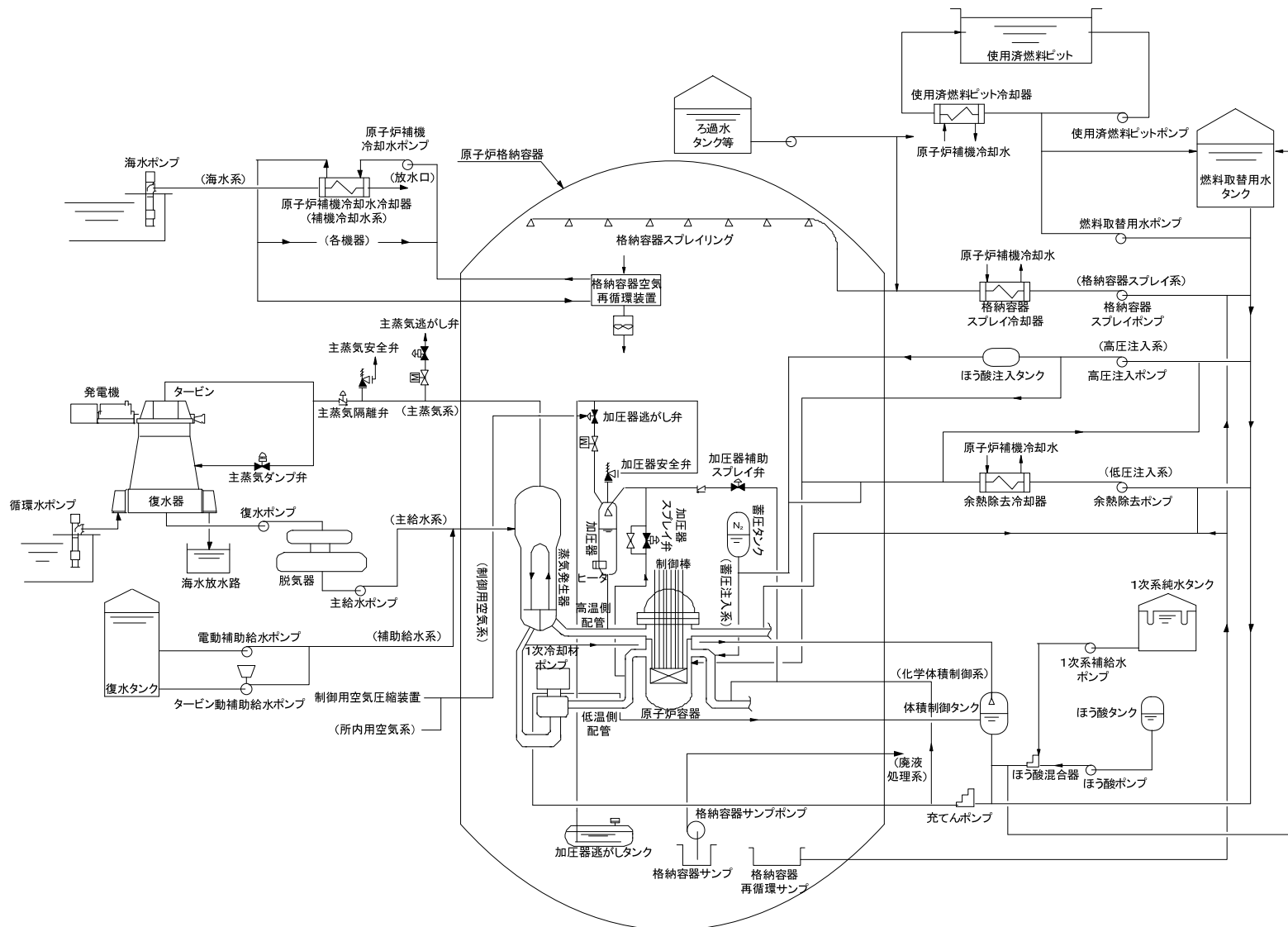
図4. 7. 1 伊方発電所第1号機基本系統図
