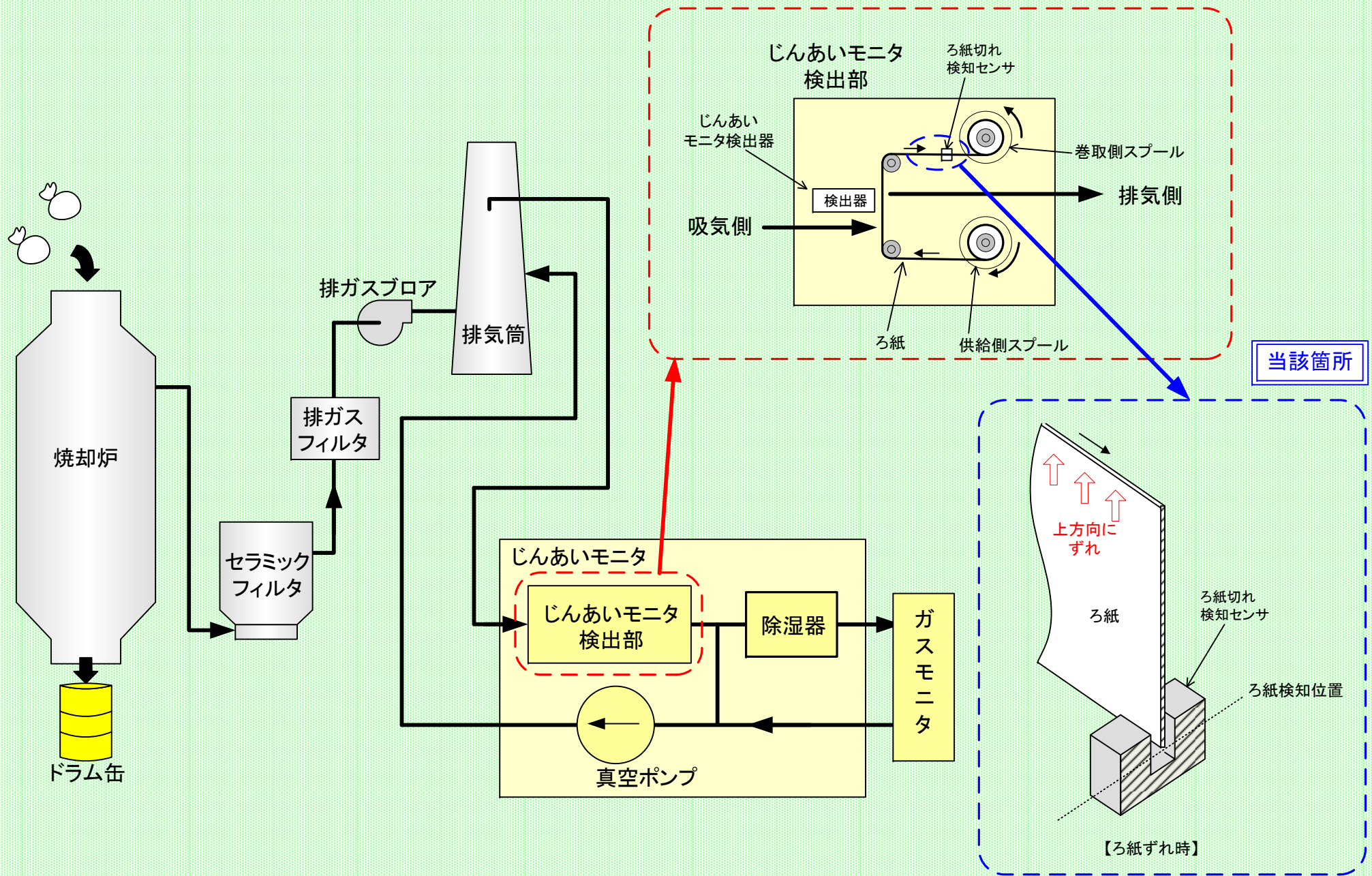
伊方発電所 雑固体焼却設備排気筒モニタ系統概略図
