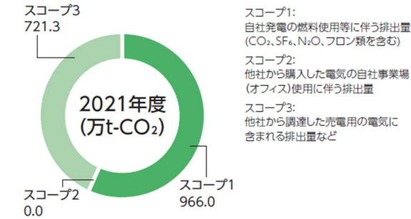
図-10 サプライチェーンにおける温室効果ガス排出量(スコープ 1, 2, 3)とスコープ 3 の内訳 (2021 年度)
