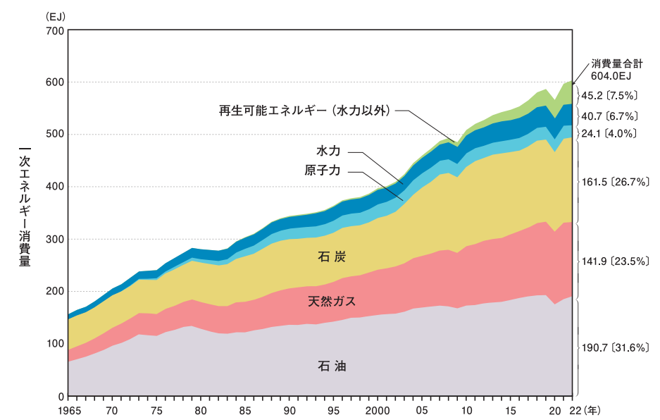
世界の一次エネルギー消費量の推移
