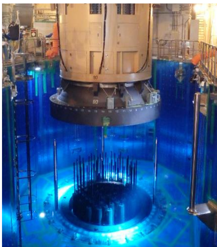
原子炉容器開放作業状況（原子炉格納容器内 3月11日撮影）
