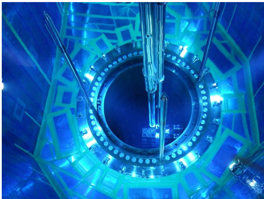
燃料装荷作業状況（原子炉格納容器内 5月4日撮影）
