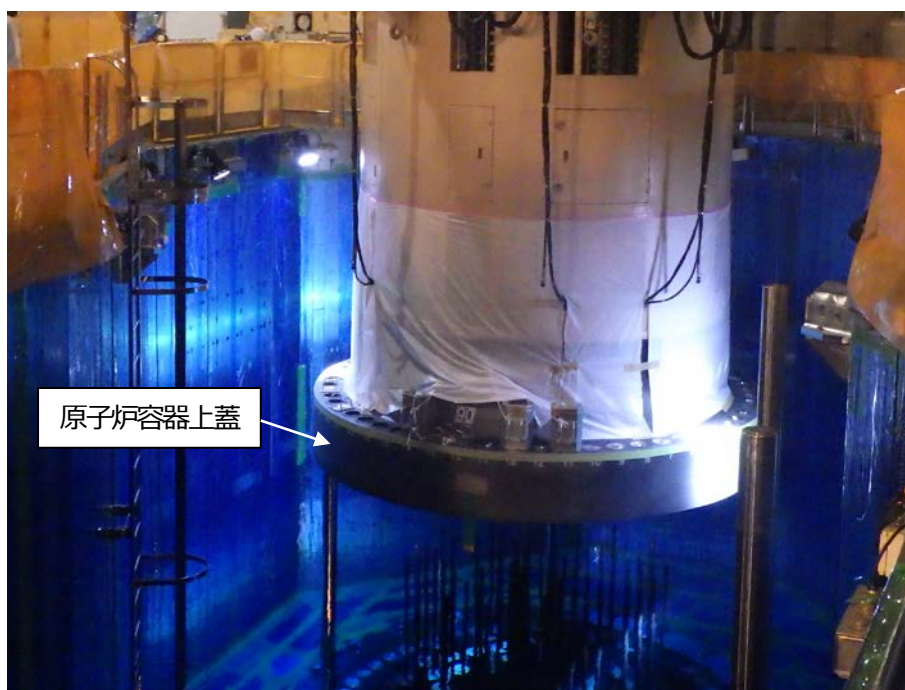
原子炉容器上蓋吊込み作業状況（原子炉格納容器内 9月14日撮影）
