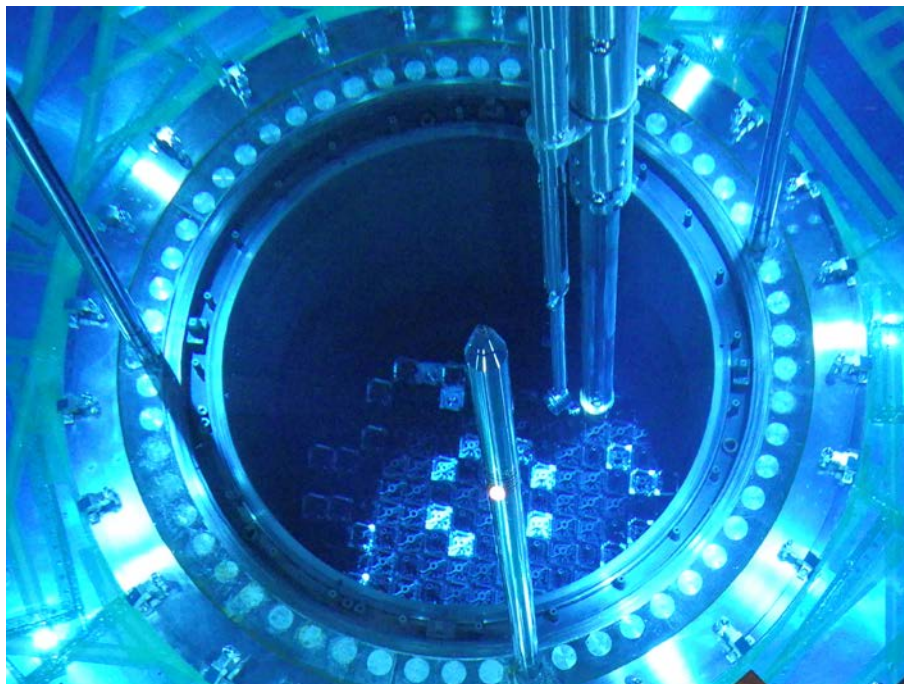
燃料装荷作業状況（原子炉格納容器内 9月12日撮影）
