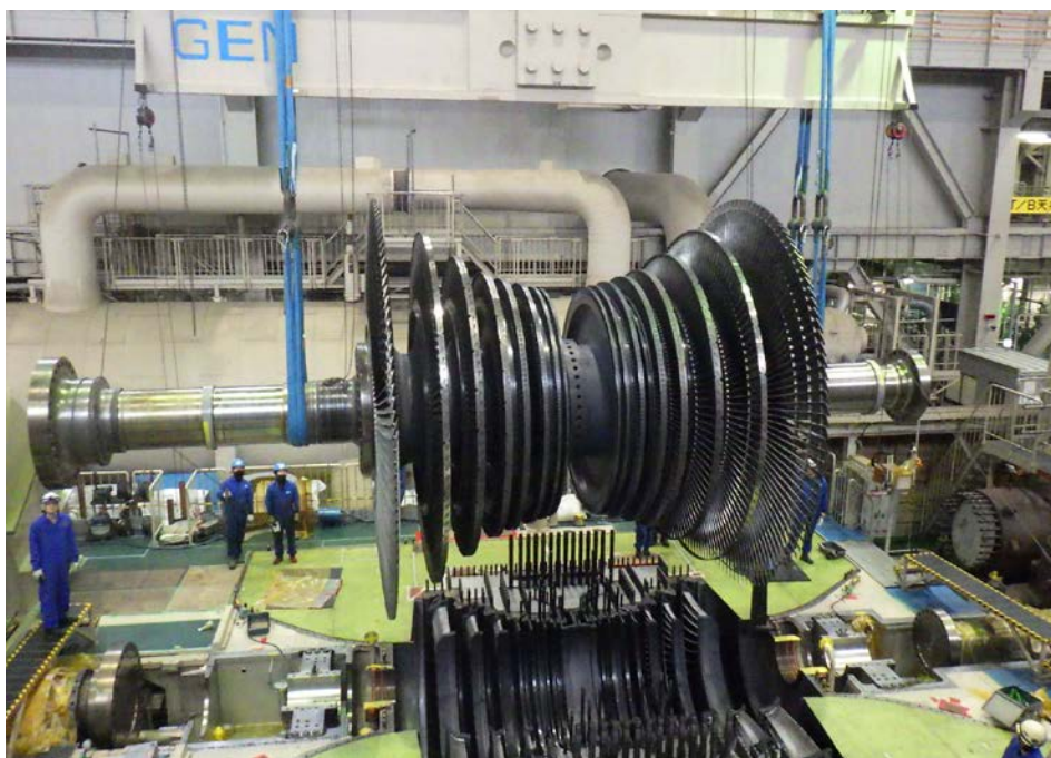
タービン点検（低圧タービンロータ吊出）作業状況（タービン建屋内 10月20日撮影）
