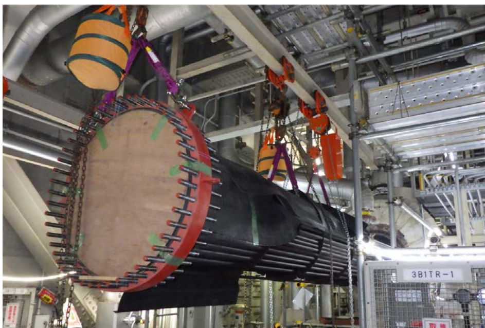
熱交換器の点検（スチームコンバータ*加熱管の取出）作業状況（タービン建屋内 10月29日撮影）
