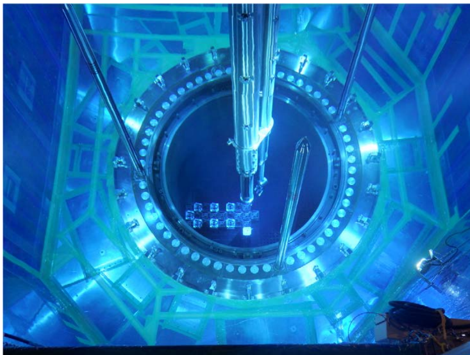
燃料装荷作業状況（原子炉格納容器内 11月29日撮影）
