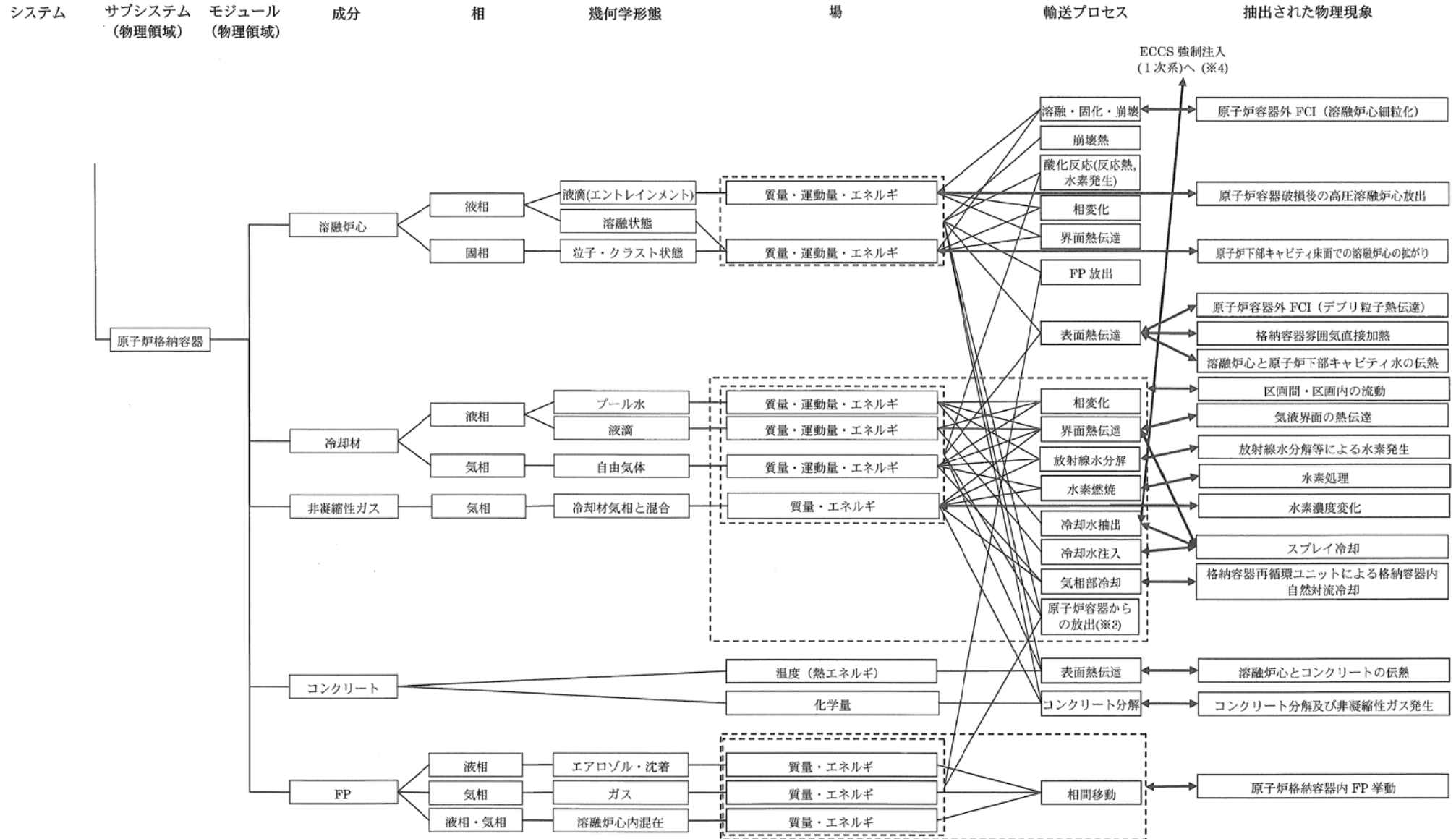
図 3-1 有効性評価における物理領域の階層化と物理現象の整理 (4/4)
