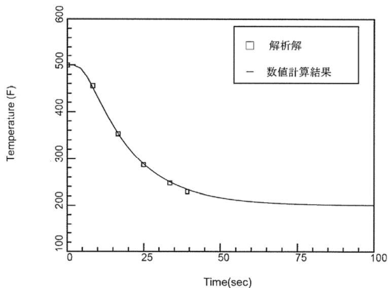
図 4-31 1次元熱伝導モデルと解析解の比較
