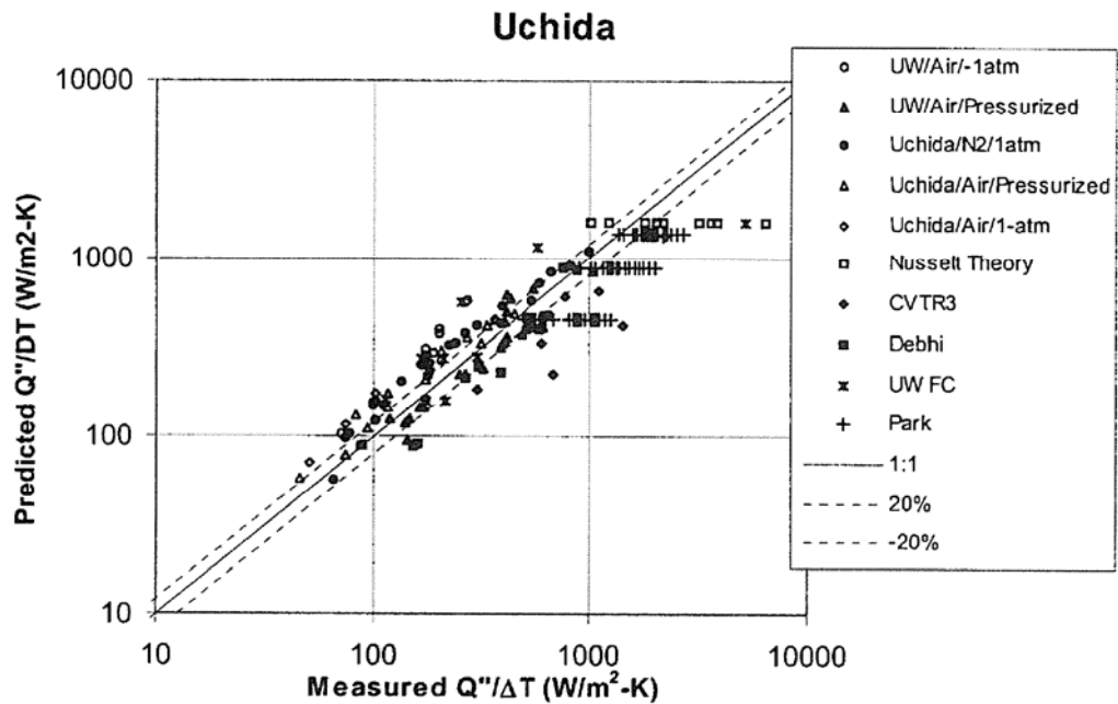
図 4-29 内田凝縮相関式の実験予測特性
