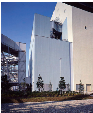
排煙脱硝装置(橘湾発電所)
