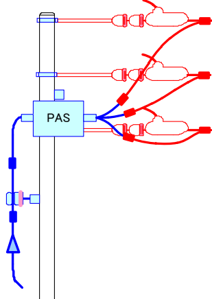
(垂直配線の例)
