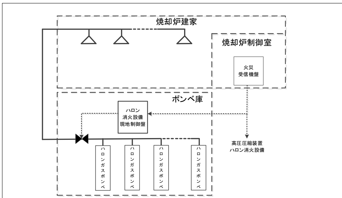
【伊方発電所焼却炉建家 ハロン消火設備概略図】
