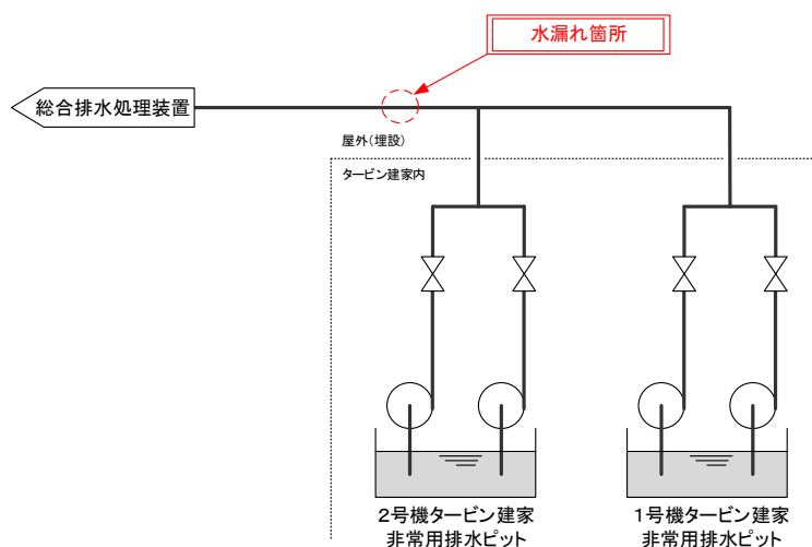
伊方発電所1、2号機 タービン建家非常用排水系統概略図
