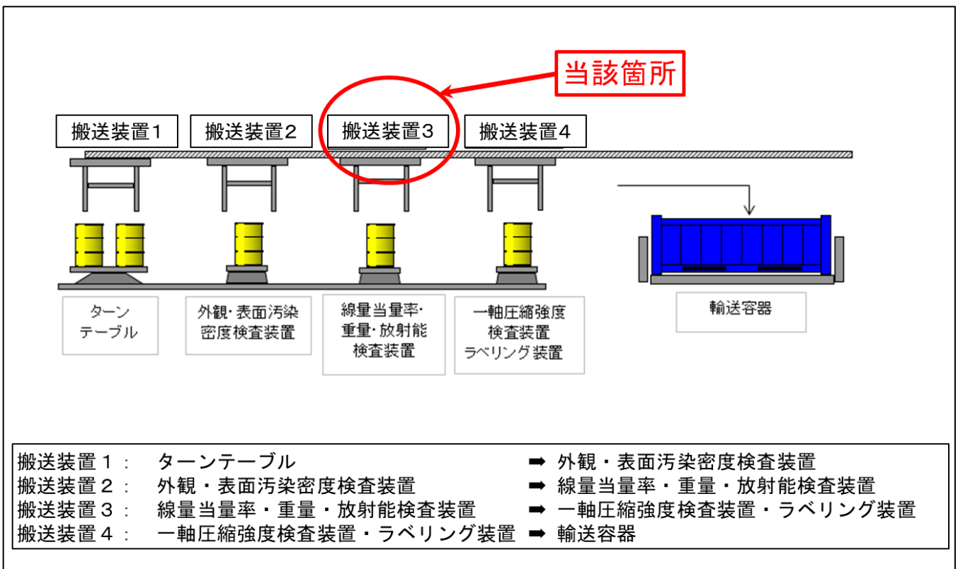
伊方発電所 低レベル放射性廃棄物搬出検査装置概略図
