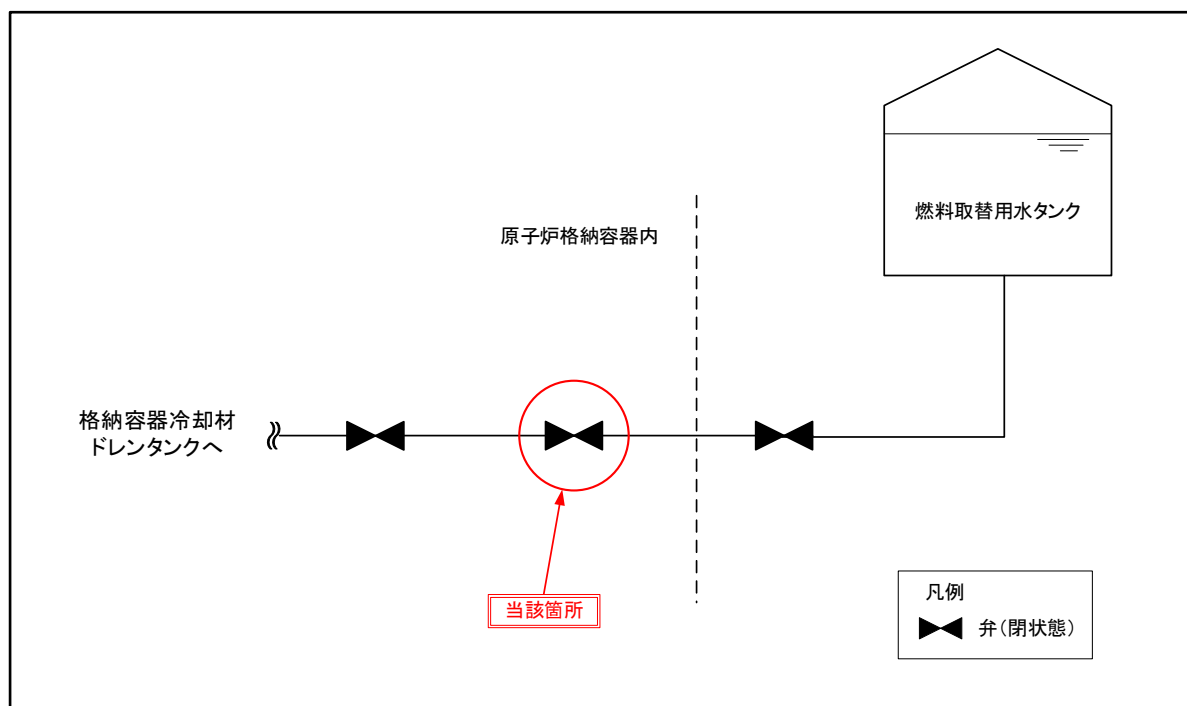
伊方発電所 1 号機 燃料取替用水系統概略図
