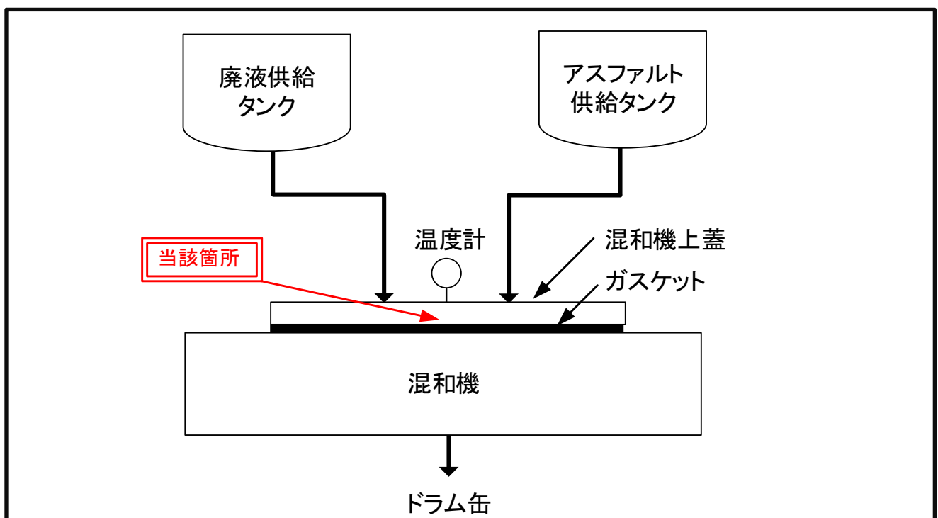
伊方発電所2号機 アスファルト固化装置 概略図
