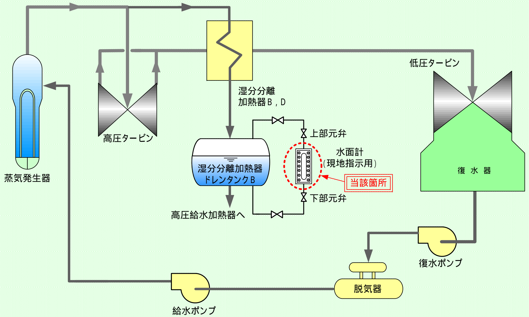
伊方発電所1号機 湿分分離加熱器ドレンタンクまわり系統概略図
