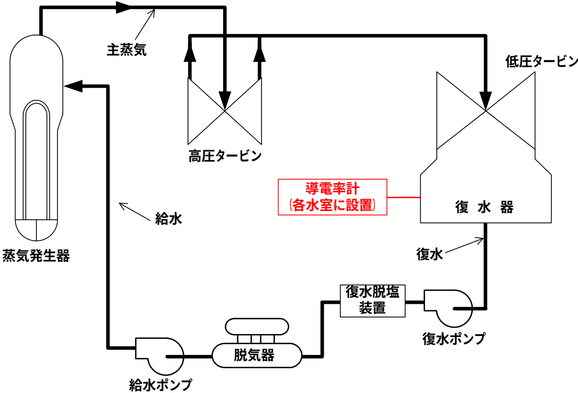
2次系系統概略図 (純水)
