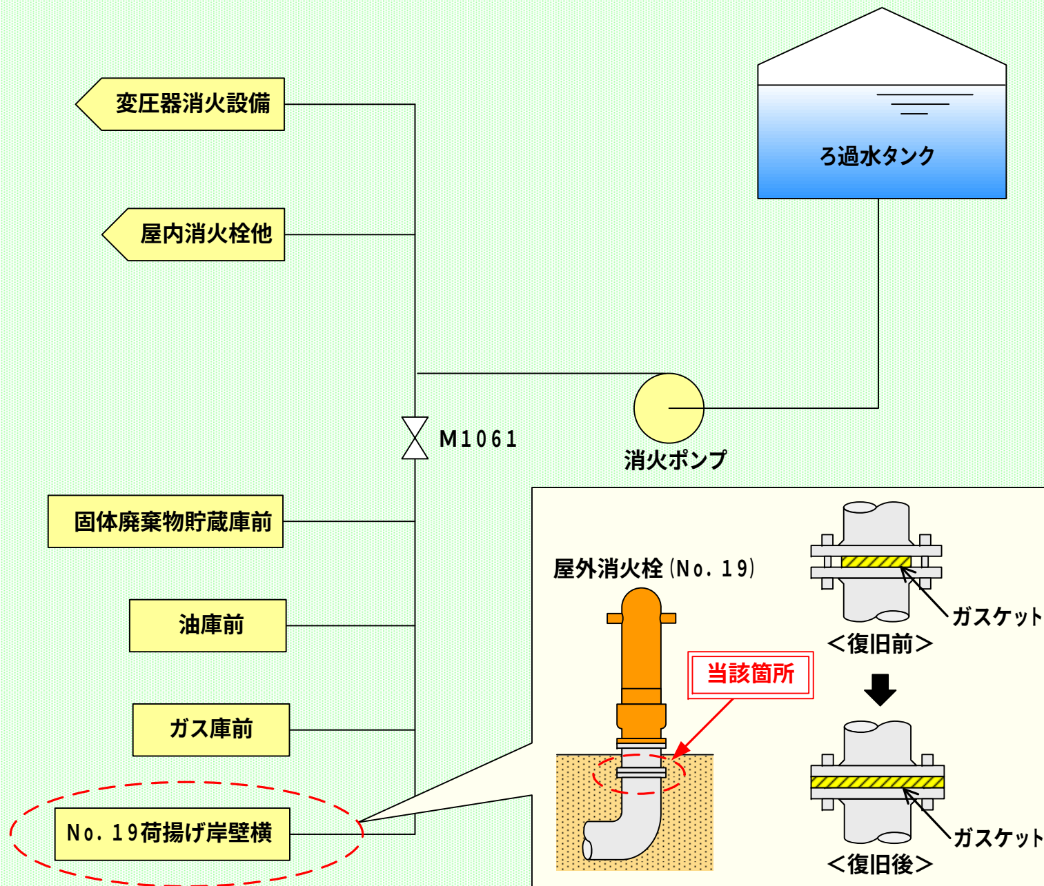
伊方発電所 屋外消火配管系統概略図
