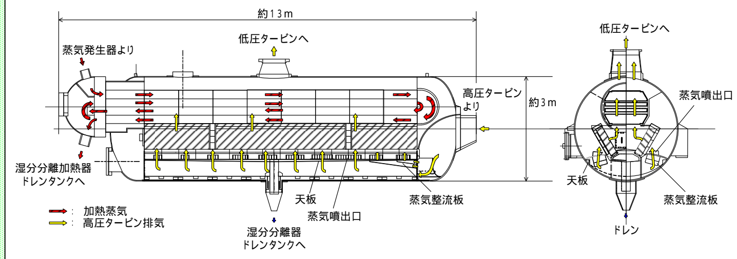
湿分分離加熱器構造図
