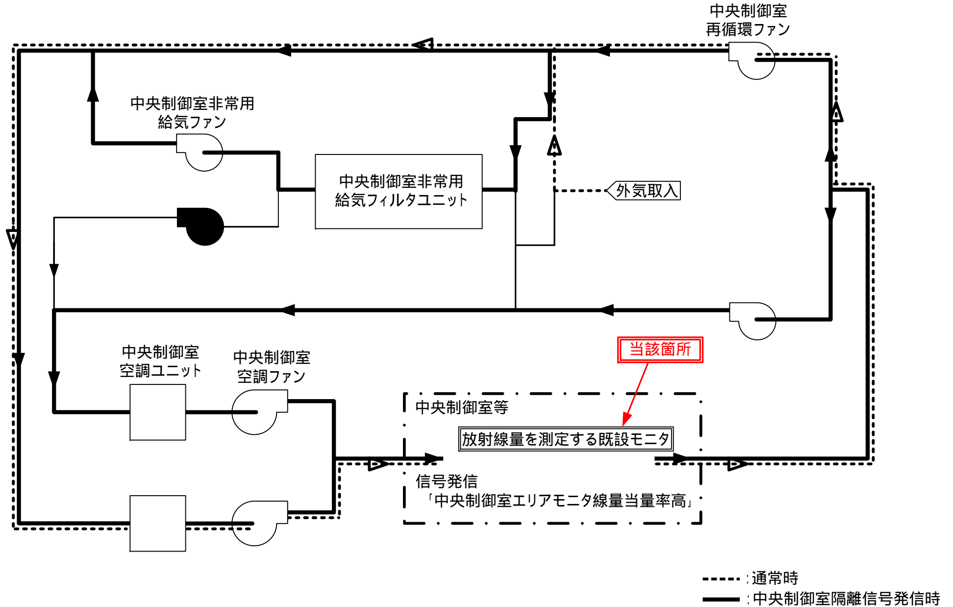
伊方発電所3号機 中央制御室非常用循環系統概略図
