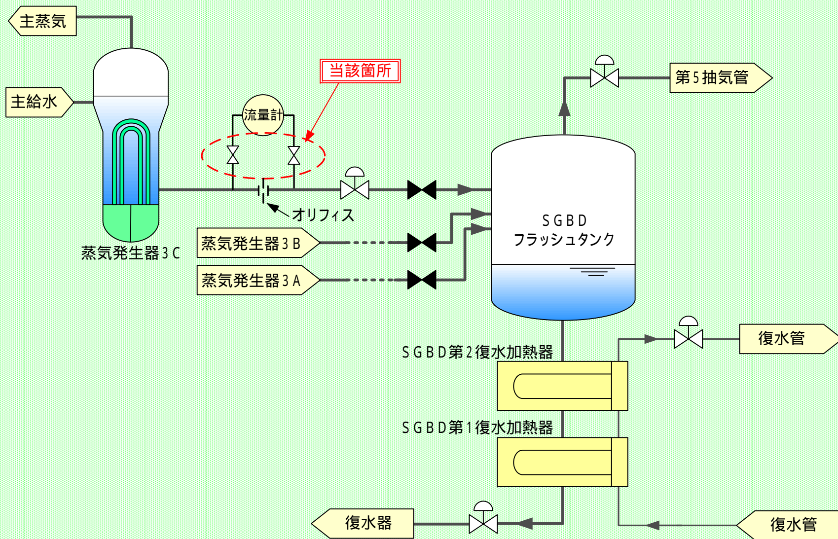
伊方発電所3号機 蒸気発生器ブローダウン(SGBD)熱回収装置概略図
