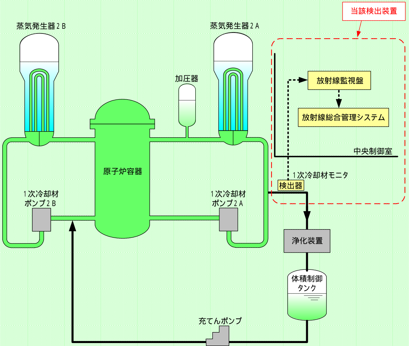
伊方発電所2号機 1次冷却材系統概略図
